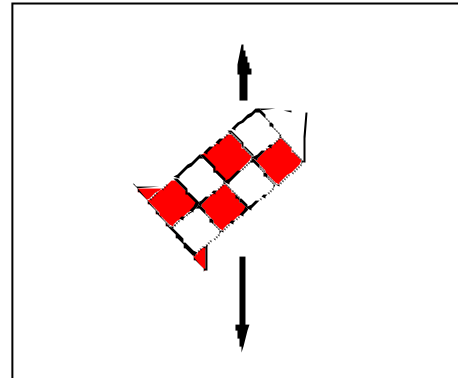
Abb. 01 Masse-Schwerkraft
